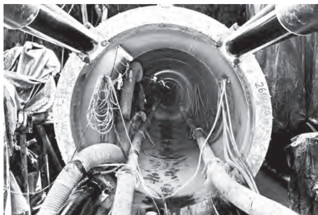
Túnel Colector San Martín
